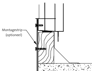
Bevestiging aan binnenzijde dakkap. (bouwkundige dakopstand)
