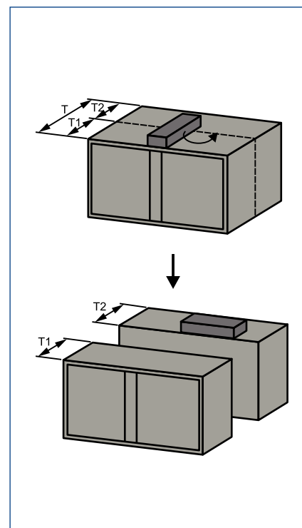
Afb. 5.7 CPL-iH-4700 evo, CPL-iH-6100 evo gedeeld, Regeling zwenkbaar
