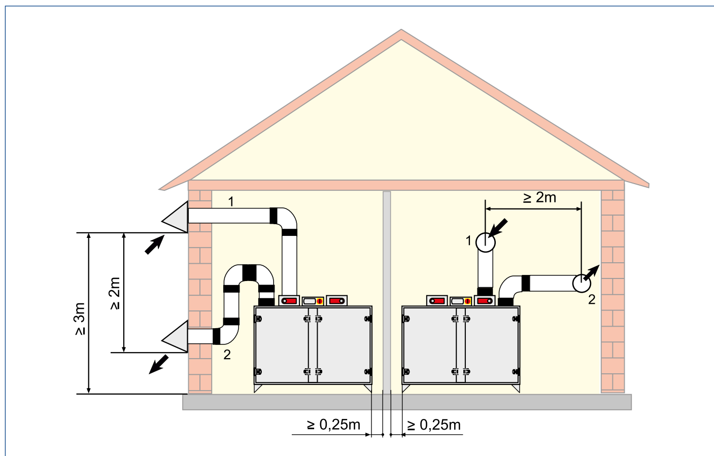
Afb. 6.1 CKL-A evo minimale afstand aanzuiging - uitblazing
