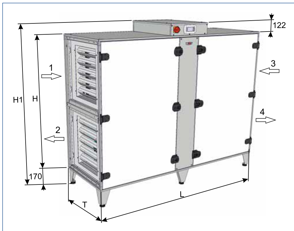
Afb. 5.6 CPL-iH evo afmetingen
