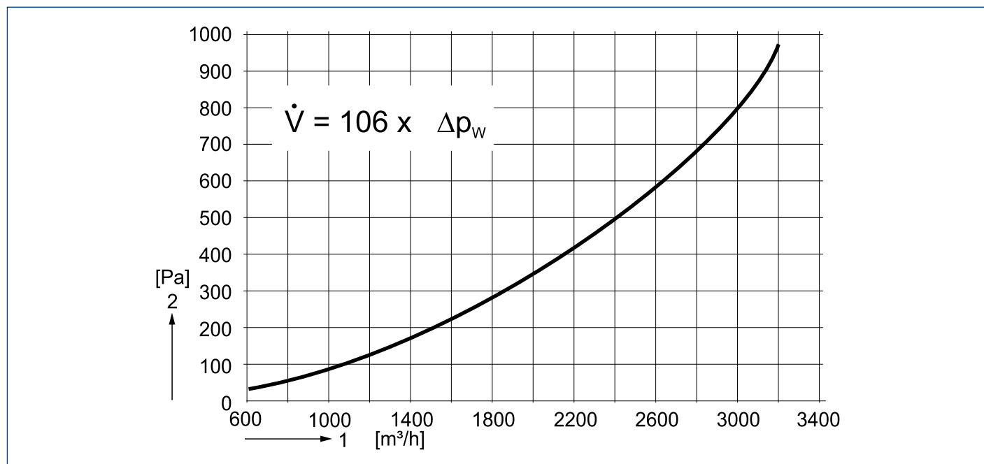
Afb. 8.4 Drukverschil CPL-3300 evo
