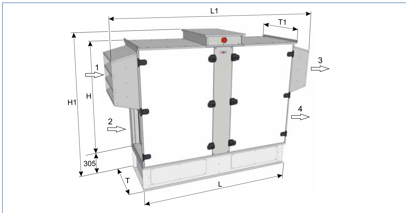
Afb. 5.9 CPL-A evo afmetingen
