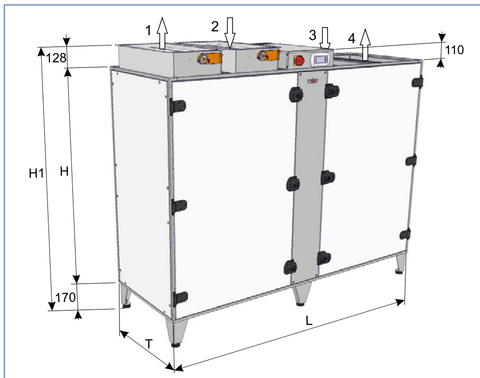
Afb. 5.2 CPL-iV evo afmetingen
