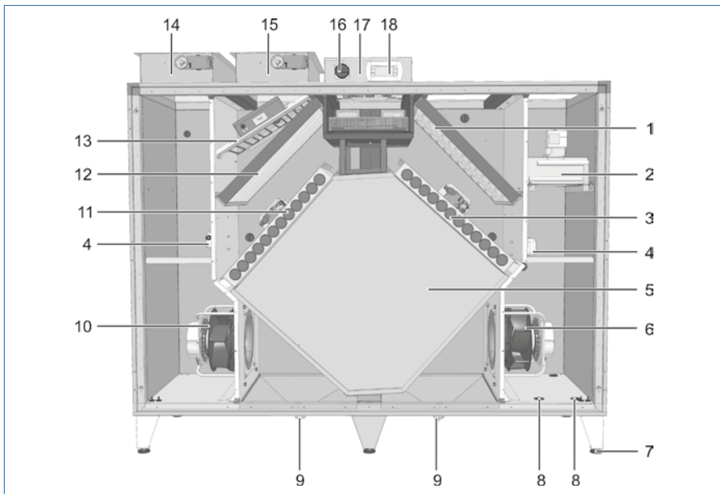
Afb. 5.8 CPL-A evo beschrijving
