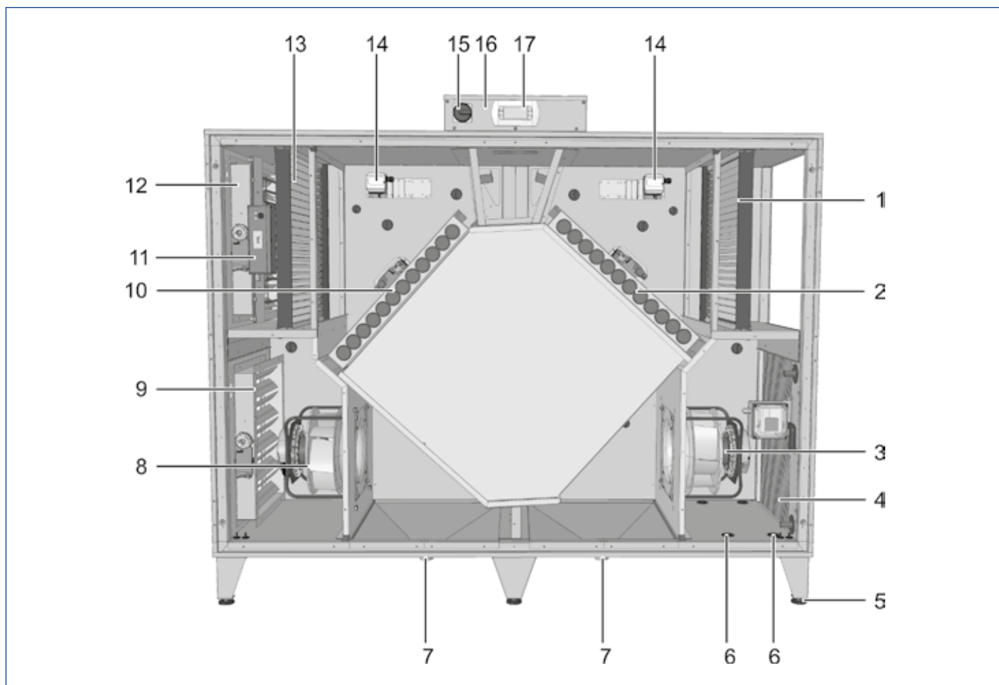
Afb. 5.5 CPL-iH evo beschrijving
