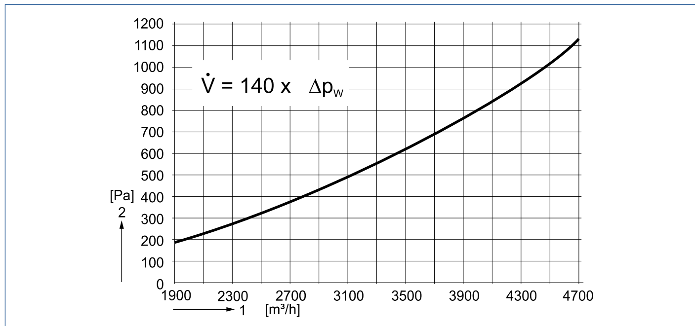
Afb. 8.5 Drukverschil CPL-4700 evo
