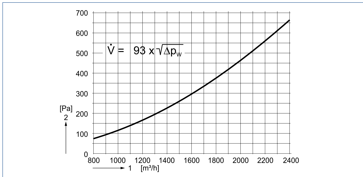
Afb. 8.3 Drukverschil CPL-1400 evo
