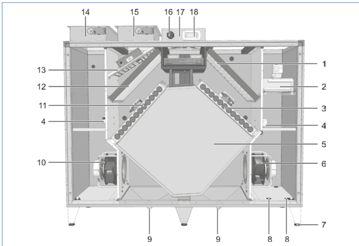
Afb. 5.1 CPL-iV evo beschrijving
