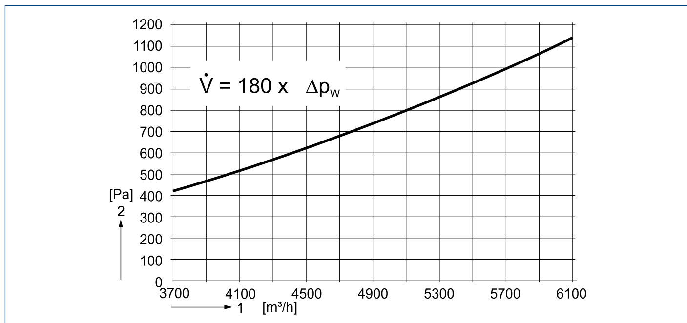
Afb. 8.6 Drukverschil CPL-6100 evo
