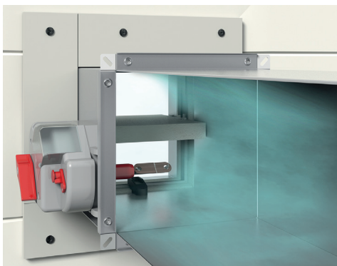
❶ De ventilatie lucht stroomt door het kanaal, de brandklep staat open (normaal bedrijf).
