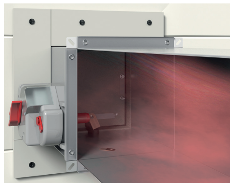
❷ Bij brand stromen hete rookgassen door het kanaal, de brandklep gaat dicht.
